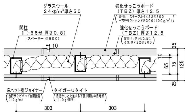
水平断面図
