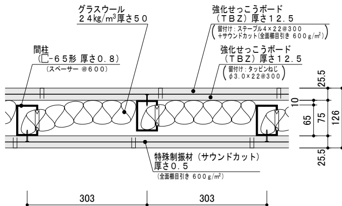
水平断面図
